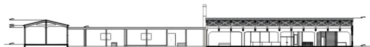
ΤΟΜΗ Β - Β
