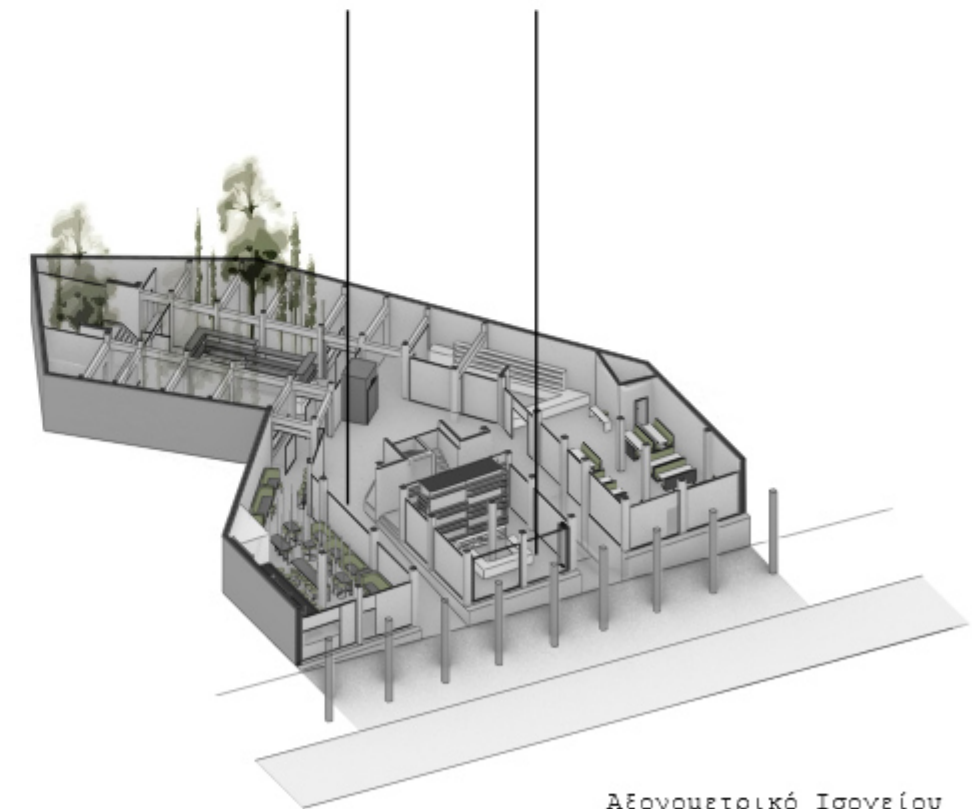
Αξονομετρικό Ισογείου
